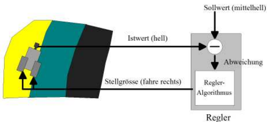
Regelungskreis
