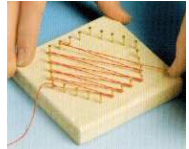
Aus Täubner, Walz: Fadengrafik
